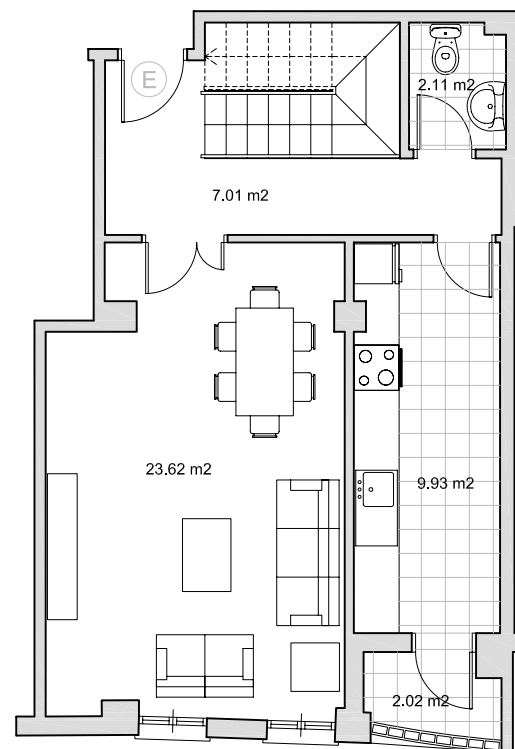
PLANTA PRIMERA
